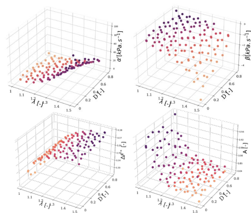
Effet de l'allongement \lambda et de l'endommagement D sur les indicateurs
