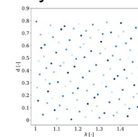
Échantillonnage quasi Monte Carlo (entraînement et validation)
