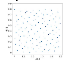
Échantillonnage quasi Monte Carlo (entraînement et validation)
