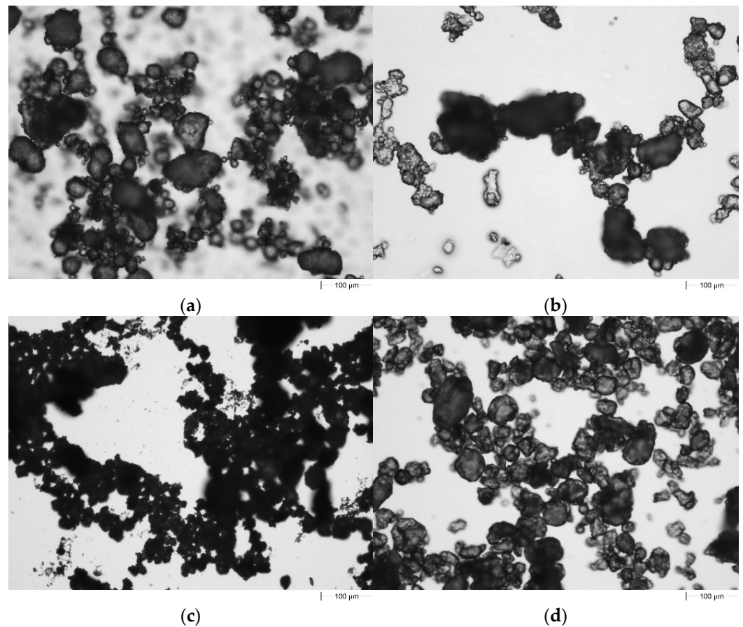
Figure 5. Microscopy observations: (a) boehmite, (b) DEPA-Al, (c) DPPA-Al, (d) DEHPA-Al.
