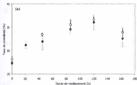
Figure 6. Évolution (a) du taux de cristallinité (b) de la température de fusion d'un composite PET/45 différents (● : FSt PET ; ○ : FSp PET ) au cours du vieillissement % en masse de fibres de verre ayant des traitements de surface
