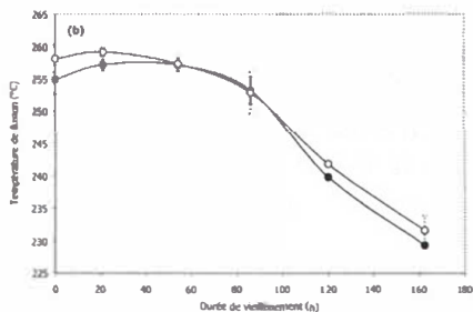
Figure 6. Évolution (a) du taux de cristallinité (b) de la température de fusion d'un composite PET/45 différents (● : FSt PET ; ○ : FSp PET ) au cours du vieillissement % en masse de fibres de verre ayant des traitements de surface
