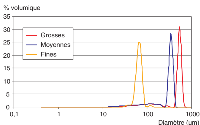
□ figure 1 Répartitions granulométriques des billes de verre.
