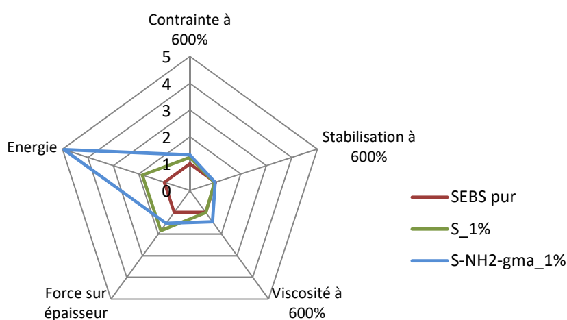
Figure 2 : Synthèse des résultats d'essais mécaniques (S_1% : SEBS chargé à 1% de sépiolite non-traitée ; S-NH2-gma_1% : SEBS chargé à 1% de sépiolite modifiée)
