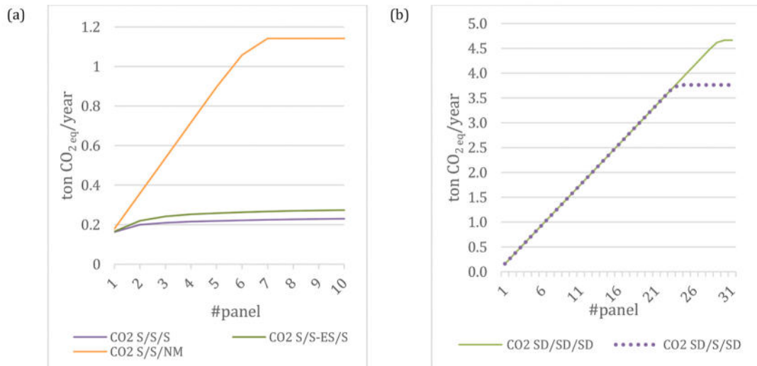
Fig. 11. (a) tCO 2eq comparison for Chilean scenarios. (b) tCO 2eq comparison for Dominican scenarios.
