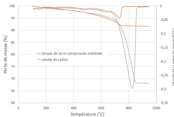
FIGURE 5. analyse thermogravimétrique
