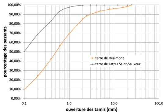
FIGURE 4. analyse granulométrique
