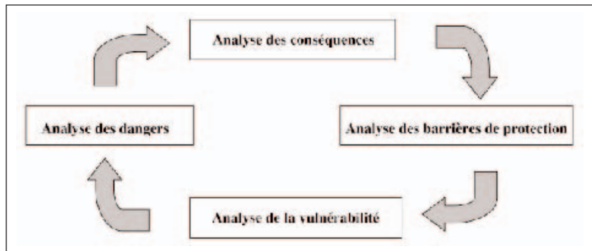
Fig. 1. - Méthode SARA.
