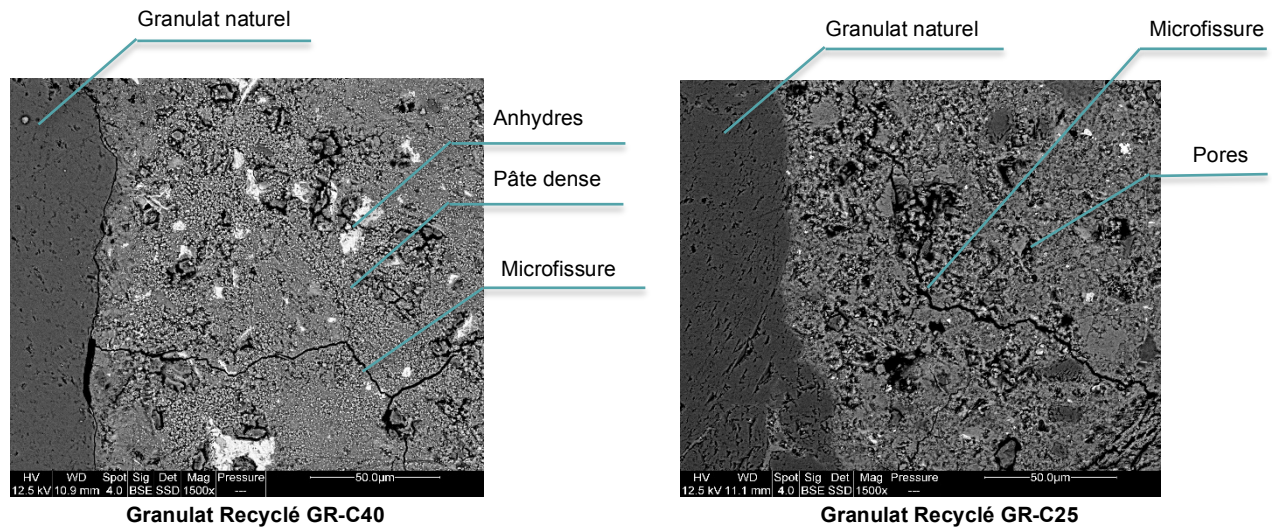
Figure 9 : Photos au Microscope Electronique à Balayage des GR
