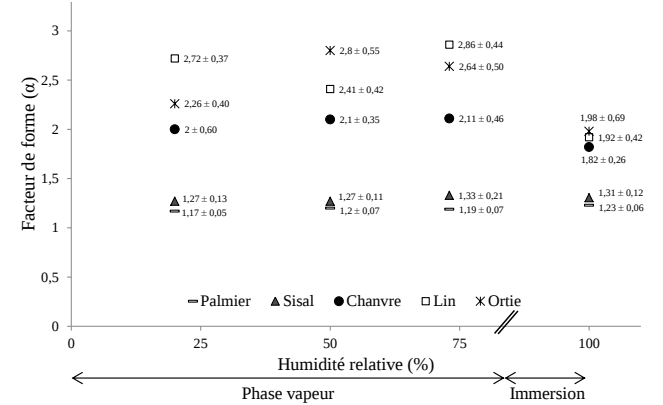
Figure 3. Evolution du facteur de forme médian \alpha en fonction de l’humidité relative à 23 °C pour les différents types de faisceaux de fibres végétales
